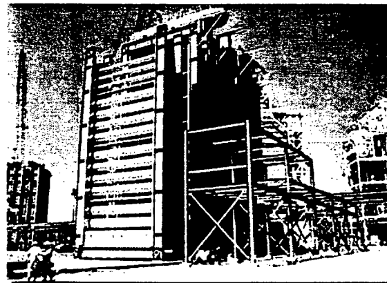
Figure 15 – Duct Burner and HRSG
