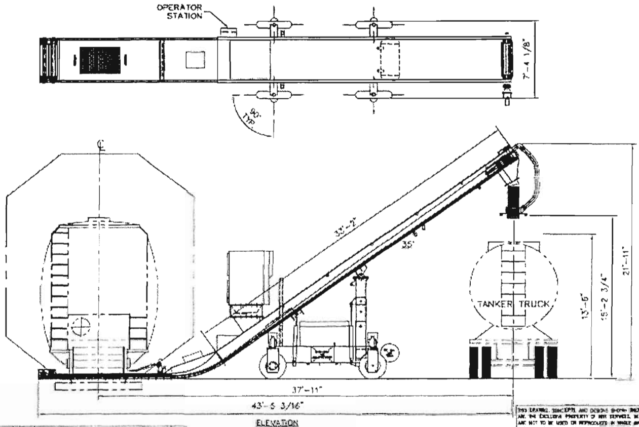
ELEVATION
