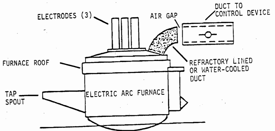
B. ELEVATION
